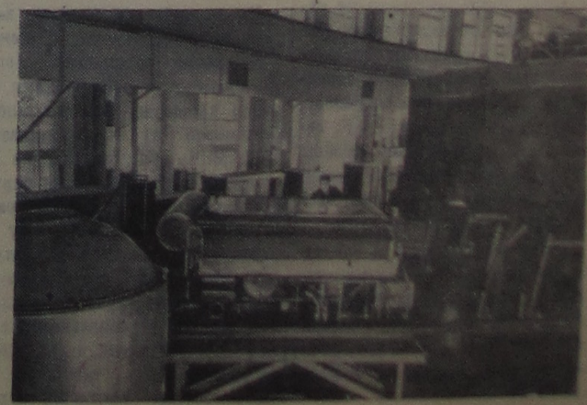
В измерительном павильоне синхрофазотрона. Большая диффузионная камера. Фото В. Шустина.
