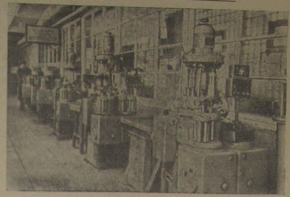
На Втором Московском часовом заводе проводится большая работа по механизации и автоматизации производства. Здесь, в частности, создается цех-автомат для изготовления основ часового механизма так называемых платин. В цехе будут установлены специальные многопозиционные агрегатные станки-автоматы, создаваемые на самом заводе. Часть этих станков уже изготовлена и работает. На снимке: участок многопозиционных агрегатных станков-автоматов, предназначенных для изготовления платин.
