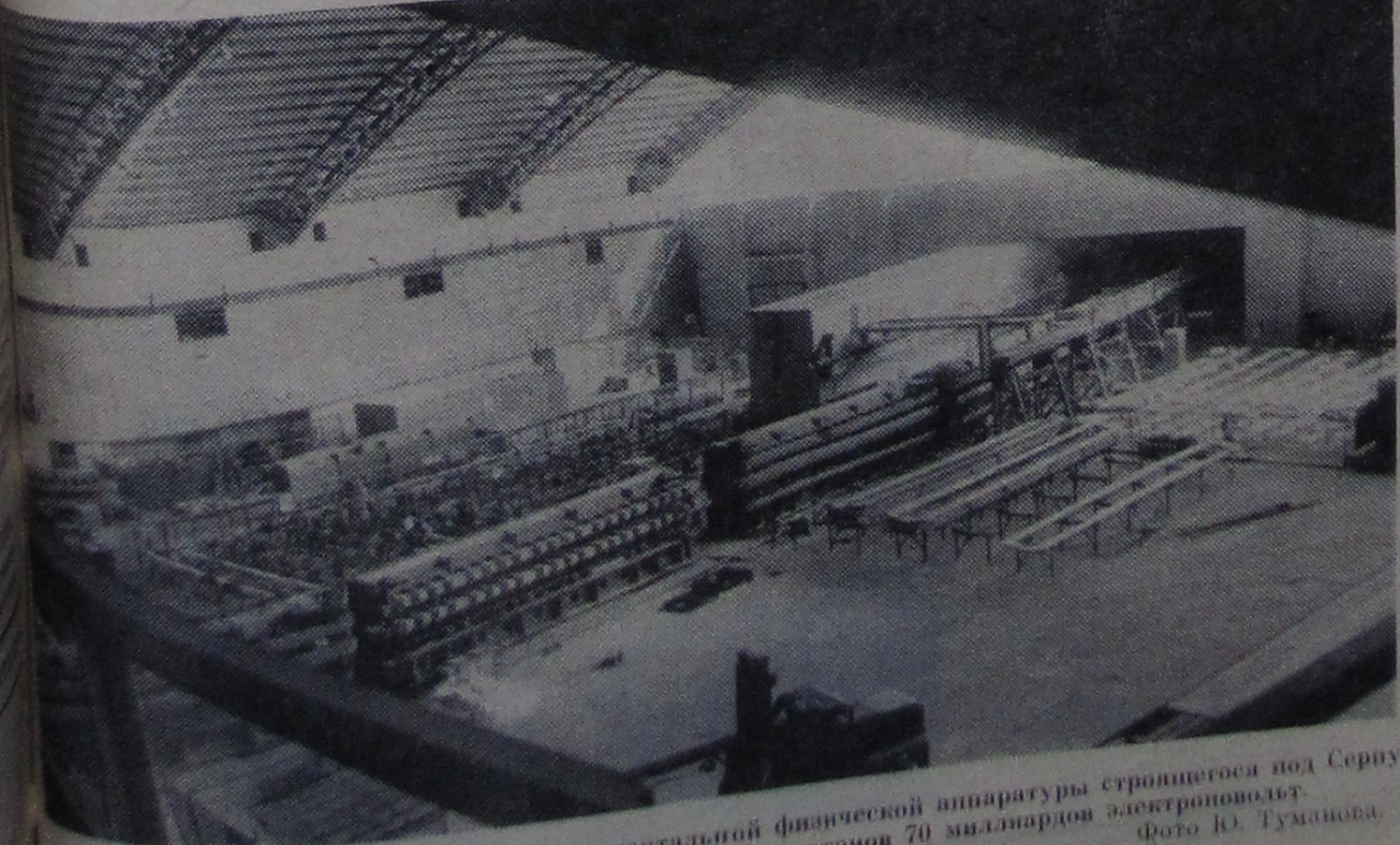
На снимке: гигантский зал для экспериментальной физической аппаратуры строящегося под Серпуховом ускорителя с энергией протонов 70 миллиардов электронвольт. Фото Ю. Туманова.
