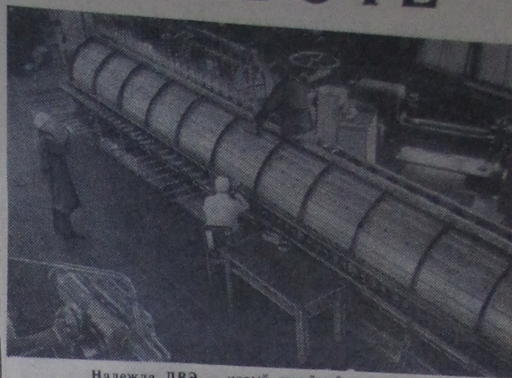
Надежда ЛВЭ — новый линейный ускоритель. Фото Ю. Туманова
